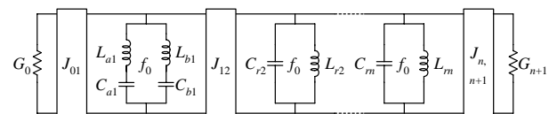
(a) Jインバータのみを用いた回路
