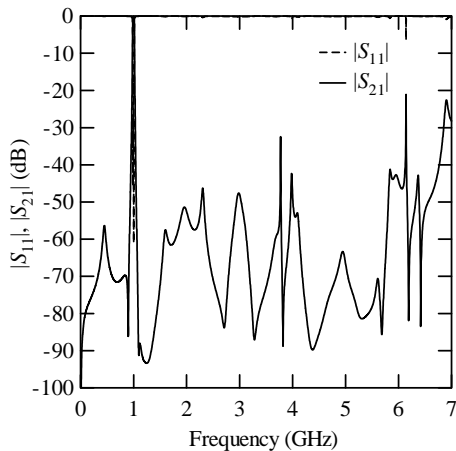
(b) 広帯域特性
