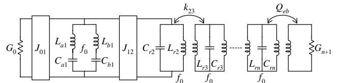
(b) Jインバータ、結合係数 k_{ij} および外部 Q を用いた回路
