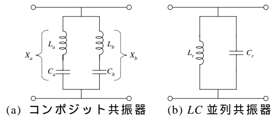
図2 共振器の等価回路
