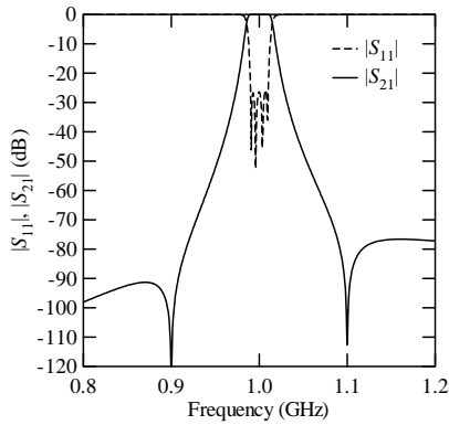
図5 4段BPF等価回路の周波数特性
