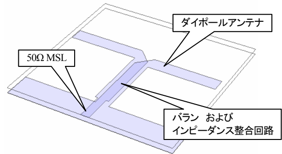
図 1 プリントダイポールアンテナ
