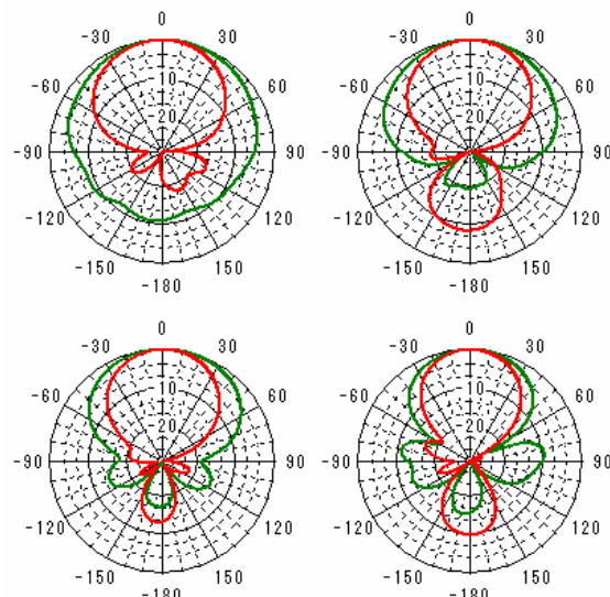
図14 放射パターン(赤:E面、緑:H面)
