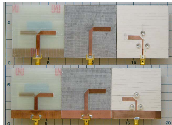
図 2 プリントダイポールアンテナ外観
