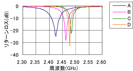
図11 リターンロス特性
