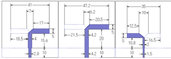
図3 プリントダイポールアンテナ寸法 左から、ガラスエポキシ、フッ素樹脂、高誘電率PP0 基板サイズは、全て60×60 (単位:mm)
